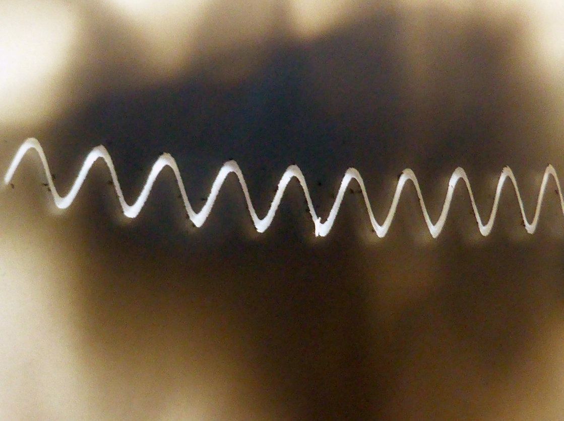
Transversalwelle
